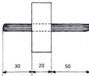
4 sz. kép A tengely beragasztása a fahengerbe (pörgettyű lendkere)
