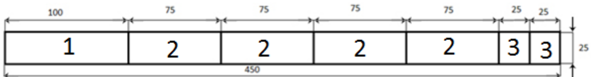
2 sz. kép Az állvány egyes részei számára szolgáló lécz
