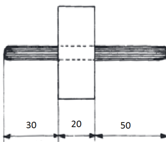
Obrázok 4 Vlepenie osky do dreveného kolieska (zotrvačníka) vĺčika
