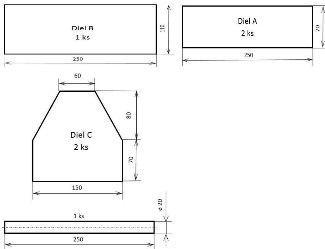
2. sz. rajz az egyes alkotórészek ábrázolása műszaki rajz segítségével
