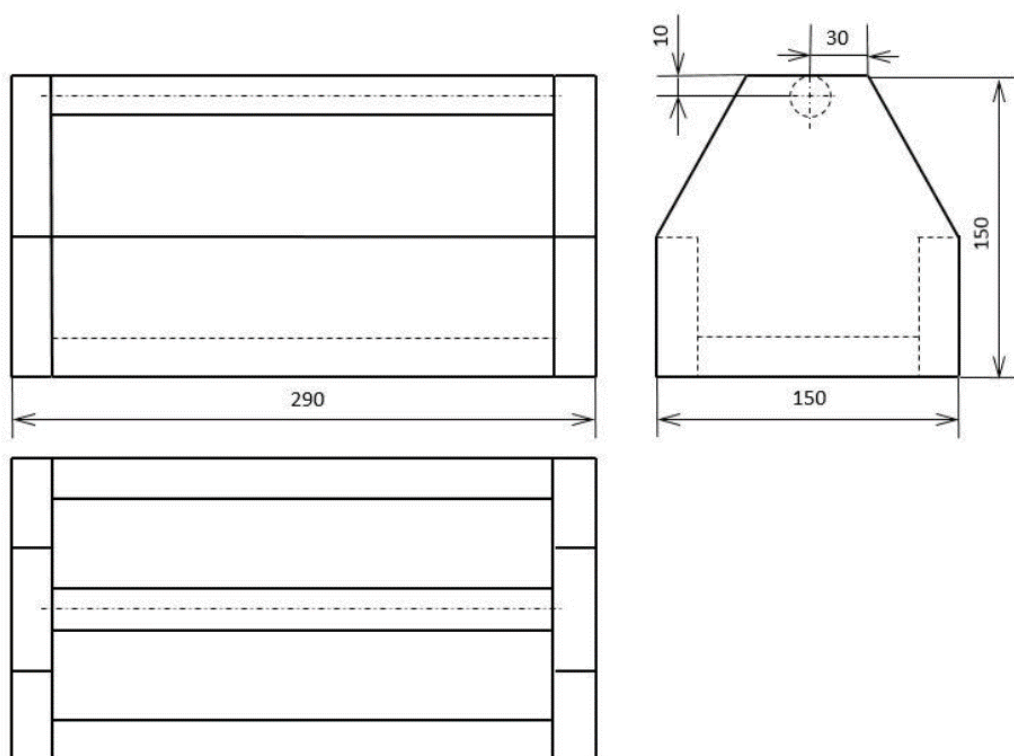
1 sz. rajz A készítmény ábrázolása derékszögű vetületben
