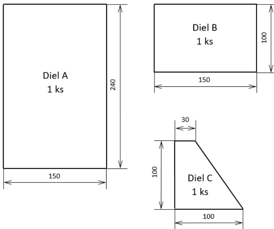
Obrázok 3 Technický náčrt jednotlivých častí výrobku
