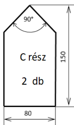
2.sz. ábra A munkadarab egyes részeinek műszaki vázlatrajza
