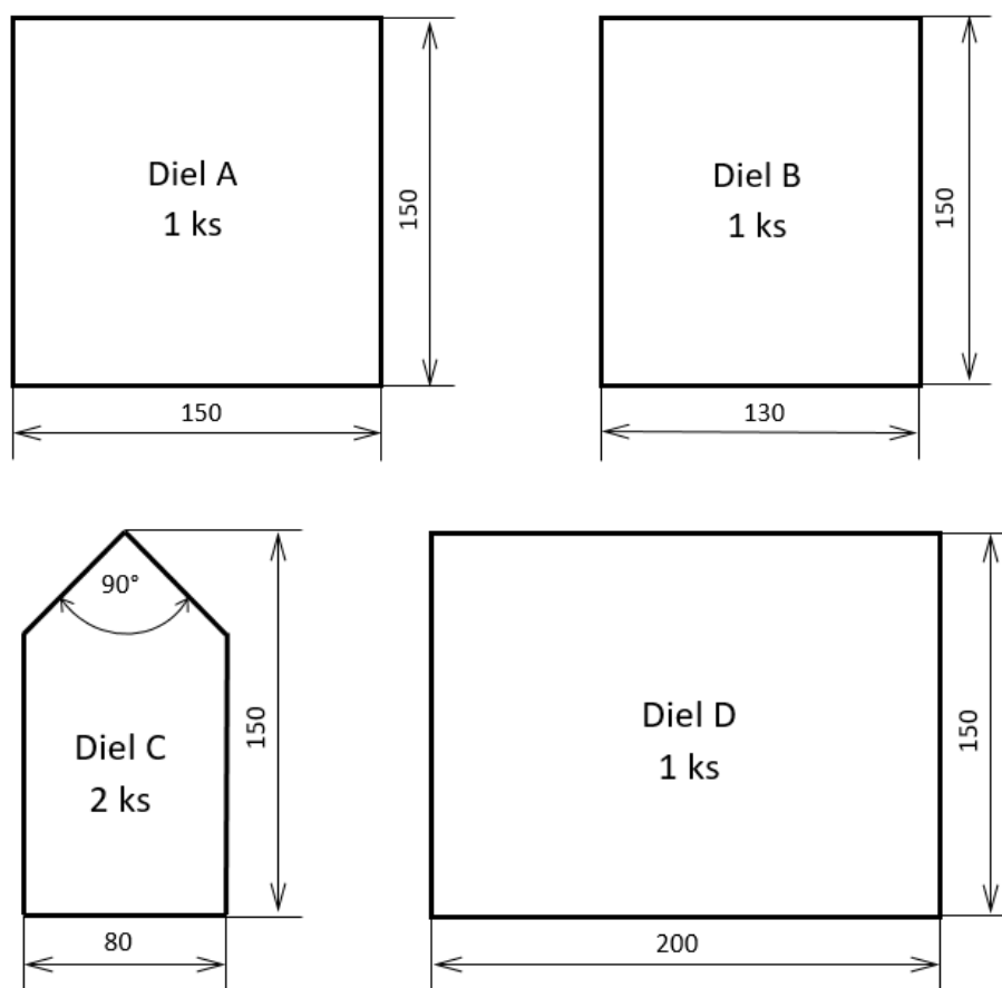
Obrázok 2 Technický náčrt jednotlivých častí výrobku
